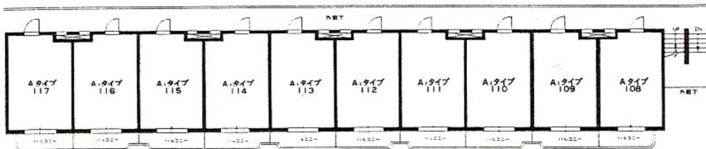
1階平面図
