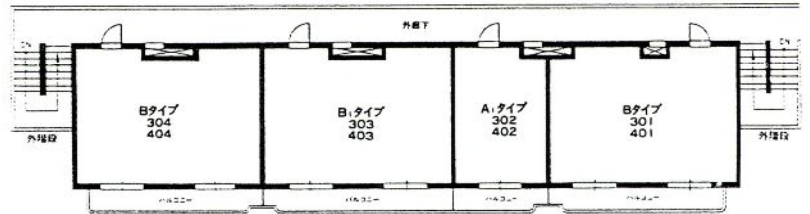
3・4階平面図
