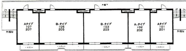
1・2階平面図
